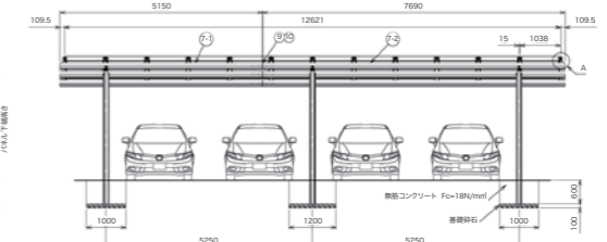
正面図 SCALE 1:100
