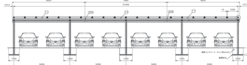
正面図 SCALE 1:100
