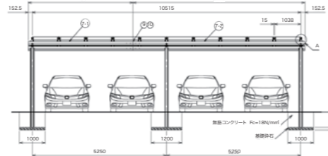
正面図 SCALE 1:100
