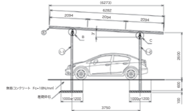
側面図 SCALE 1:100
