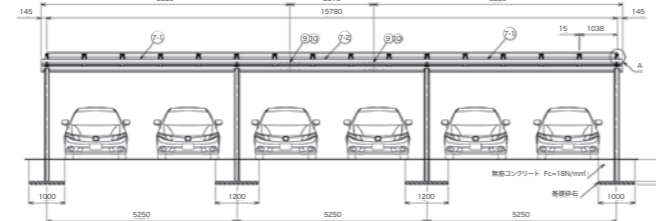
正面図 SCALE 1:100
