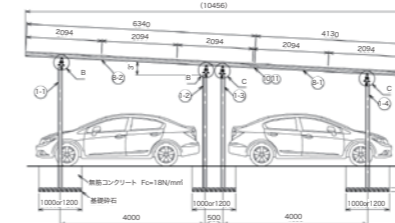
側面図 SCALE 1:100
